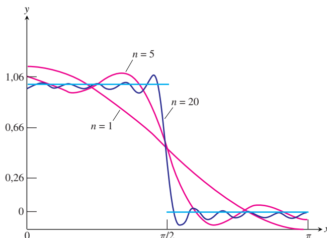
ΣΧΗΜΑ 8.29 Προσεγγίσεις με σειρά Fourier συνημιτόνων της συνάρτησης του Παραδείγματος 1 για n (πλήθος όρων) ίσο με 1, 5, και 20. Καθώς το n αυξάνεται, οι προσεγγίσεις Fourier τείνουν στις τιμές της f(x) . Στο σημείο ασυνέχειας x = \pi/2 , όλες οι συνημιτονικές προσεγγίσεις Fourier διέρχονται από το μέσον της ασυνέχειας, παίρνοντας την τιμή y = 0,5 .
