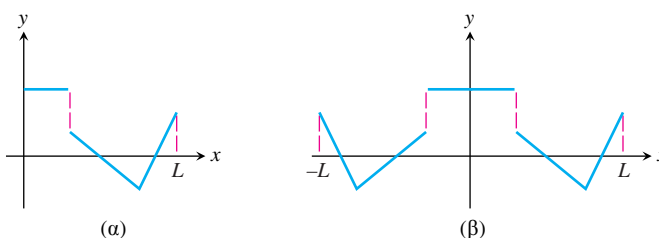
ΣΧΗΜΑ 8.26 (α) Η αρχική τμηματικά συνεχής συνάρτηση f ορίζεται στο μη συμμετρικό διάστημα 0 < x < L . (β) Η άρτια επέκταση της f στο διάστημα -L < x < L .
