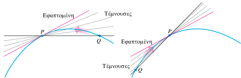
ΣΧΗΜΑ 1.60 Δυναμική ερμηνεία της έννοιας της εφαπτομένης.
