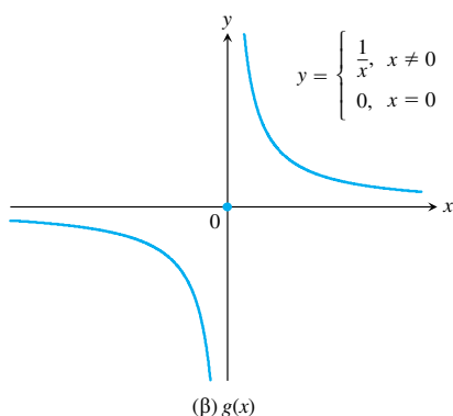
ΣΧΗΜΑ 1.8 Οι συναρτήσεις του Παραδείγματος 7.
