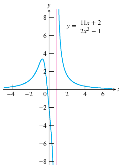
ΣΧΗΜΑ 1.28 Γραφική παράσταση της συναρτήσεως του Παραδείγματος 4. Η καμπύλη τείνει στον άξονα x καθώς το |x| αυξάνεται.
