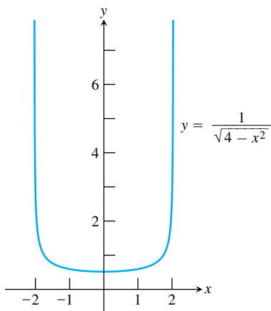
ΣΧΗΜΑ 13 (α) Αποτυχημένη σχεδίαση με υπολογιστή. (β) Μια ακριβέστερη γραφική παράσταση της συνάρτησεως y = 1/\sqrt{4-x^2} . (Παράδειγμα 3)
