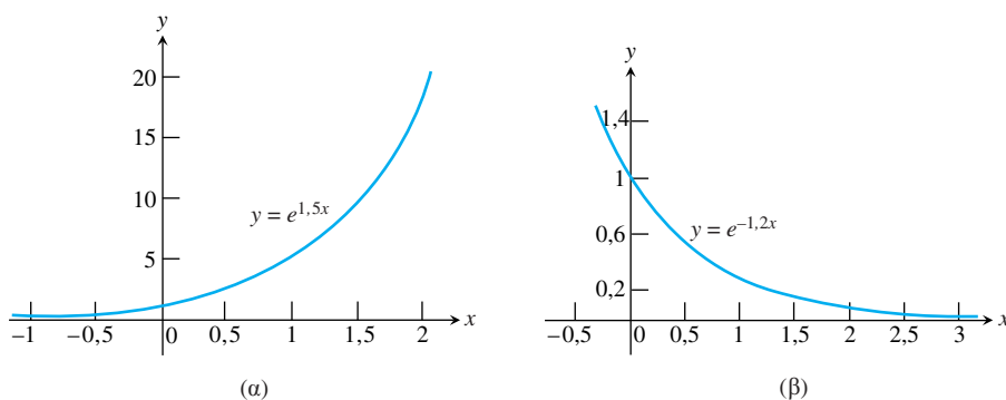
ΣΧΗΜΑ 28 Γραφήματα (α) εκθετικής αύξησης, k = 1,5 > 0 και (β) εκθετικής μείωσης, k = -1,2 < 0 .
