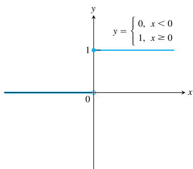
ΣΧΗΜΑ 1.8 Οι συναρτήσεις του Παραδείγματος 7.
