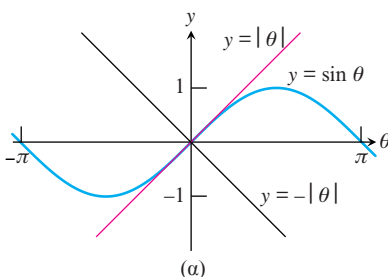
ΣΧΗΜΑ 1.19 Το θεώρημα «σάντουιτς» επαληθεύει ότι
