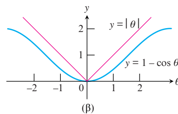
ΣΧΗΜΑ 1.19 Το θεώρημα «σάντουιτς» επαληθεύει ότι
