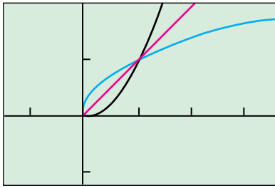
ΣΧΗΜΑ 60 Παραμετρικές γραφικές παραστάσεις της συνάρτησης f(x) = x^2, x \geq 0 , της αντίστροφής της, και της ευθείας y = x .
