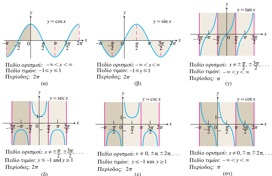
ΣΧΗΜΑ 39 Γραφικές παραστάσεις των συναρτήσεων (α) συνημιτόνου, (β) ημιτόνου, (γ) εφαπτομένης, (δ) τέμνουσας, (ε) συντέμνουσας, και (στ) συνεφαπτομένης, έναντι του ακτινίου μέτρου.
