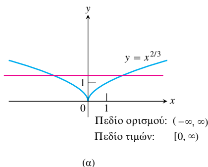
ΣΧΗΜΑ 31 (α) Το γράφημα της f(x) = x^{2/3} και μια οριζόντια ευθεία. (β) Το γράφημα της g(x) = \sqrt{x} και μια οριζόντια ευθεία. (Παράδειγμα 1)
