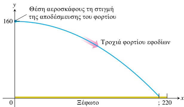
ΣΧΗΜΑ 61 Η τροχιά του φορτίου εφοδίων που έριξε το αεροσκάφος του Παραδείγματος 7.
