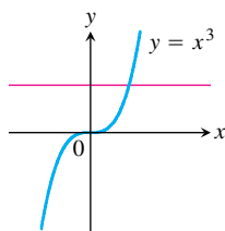
1-1: Το γράφημα τέμνει κάθε οριζόντια ευθεία μία μόνο φορά.
