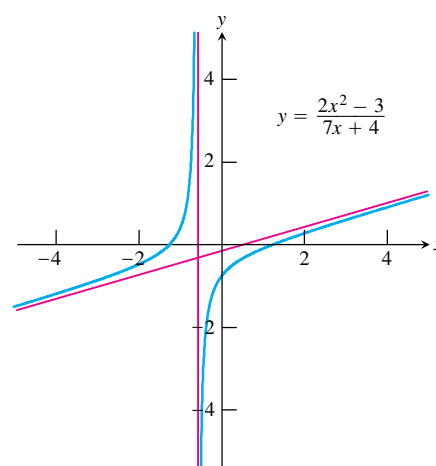
ΣΧΗΜΑ 1.29 Η συνάρτηση του Παραδείγματος 5(α).
