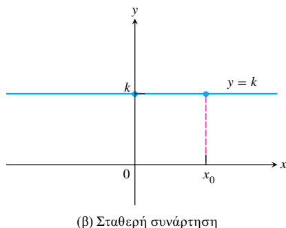
ΣΧΗΜΑ 1.7 Οι συναρτήσεις του Παραδείγματος 6.
