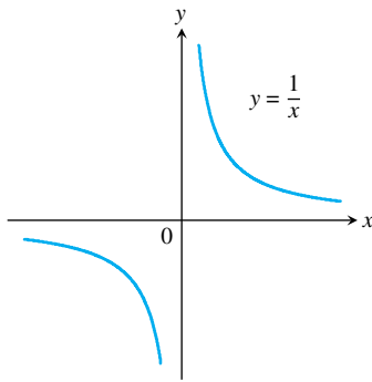
ΣΧΗΜΑ 1.51 Η συνάρτηση y = 1/x είναι συνεχής για κάθε x εκτός για x = 0 , όπου παρουσιάζει σημειακή ασυνέχεια. (Παράδειγμα 5)
