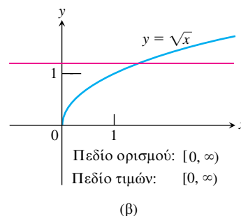
ΣΧΗΜΑ 31 (α) Το γράφημα της f(x) = x^{2/3} και μια οριζόντια ευθεία. (β) Το γράφημα της g(x) = \sqrt{x} και μια οριζόντια ευθεία. (Παράδειγμα 1)
